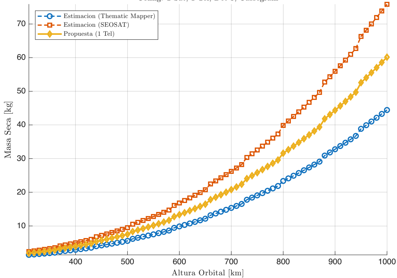
Comparativa de Masa Seca vs. Altura Config: 2 Sat, 1 Tel, Det 3, Cassegrain
